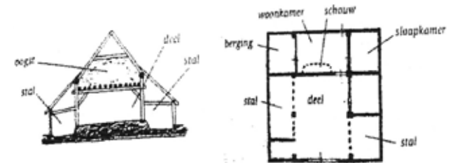
Schets van een hallehuisboerderij
